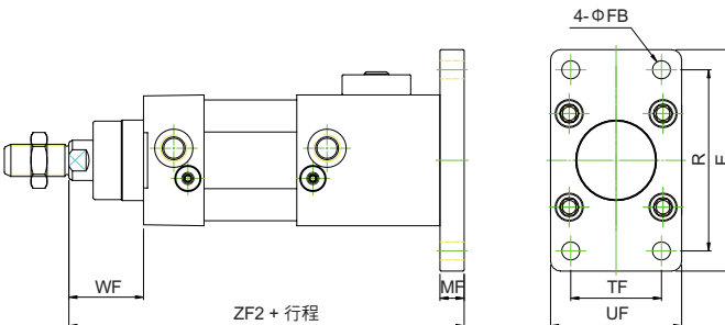
FB 複動尾端防落型 / 配件尺寸
