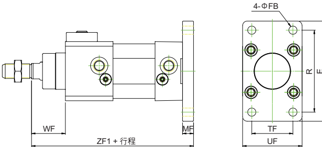
FB 複動軸端防落型 / 配件尺寸
