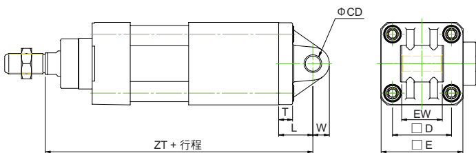
CA 複動尾端防落型 / 配件尺寸
