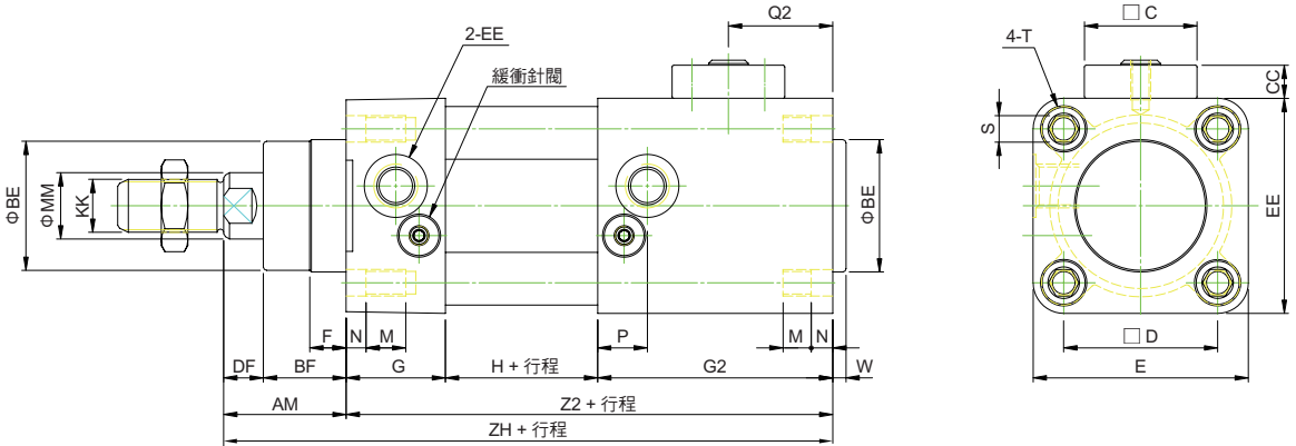
AZK 複動尾端防落型 / 外型尺寸
