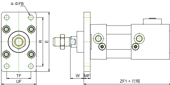
FA 複動尾端防落型 / 配件尺寸
