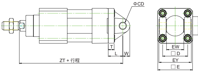
CB 複動尾端防落型 / 配件尺寸
