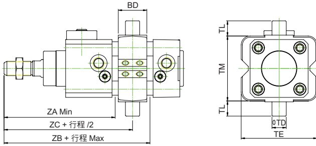
TC 複動尾端防落型 / 配件尺寸
