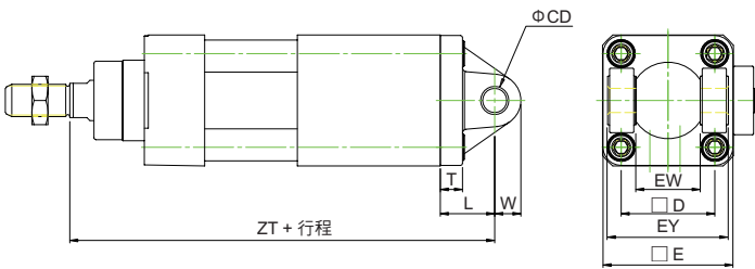
CB 複動尾端防落型 / 配件尺寸
