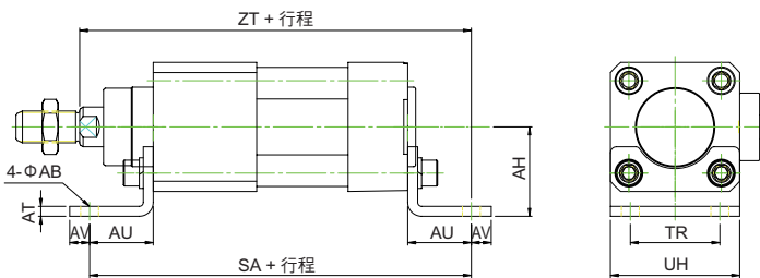
LB 複動尾端防落型 / 配件尺寸
