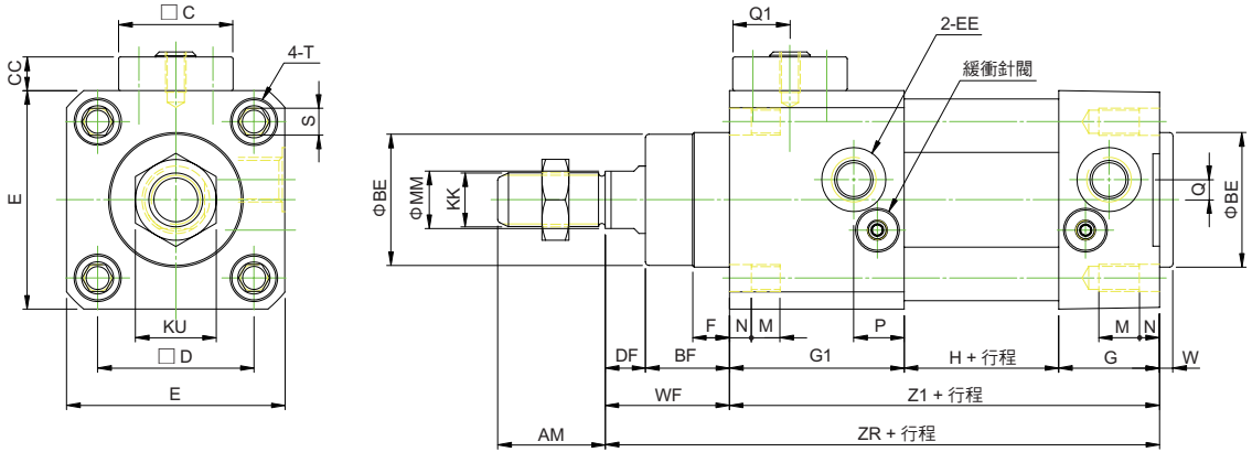
AZK 複動尾端防落型 / 外型尺寸
