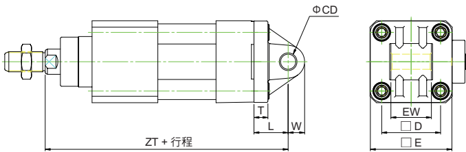
CA 複動尾端防落型 / 配件尺寸
