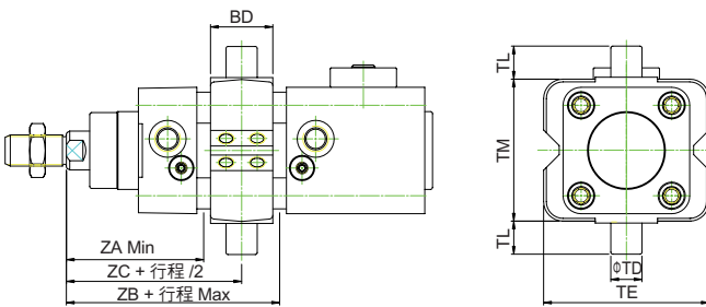
TC 複動尾端防落型 / 配件尺寸
